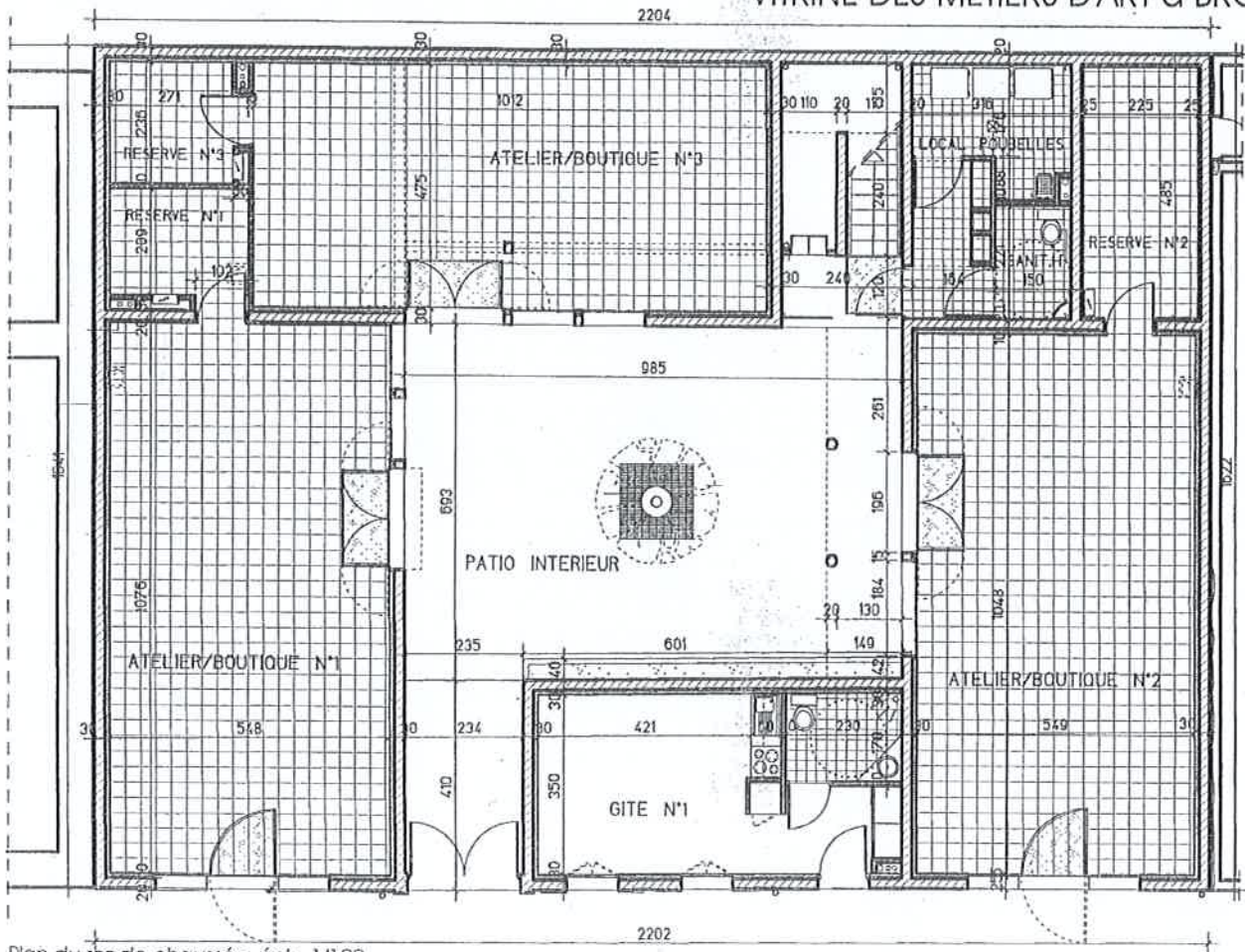
Plan du rez-de-chaussée, éch. 1/100
